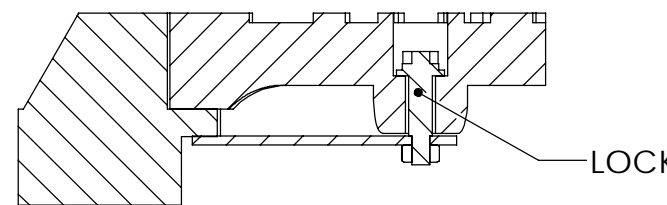
SECTION B-B SCALE 1 : 4
